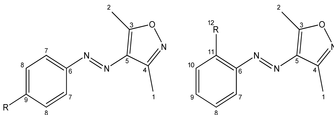
Figura 5: Estructura de isoxazoles sustituidos en posición para y del ácido 2-((3,5-dimetilisoxazol-4-il)diazenil)benzoico.
